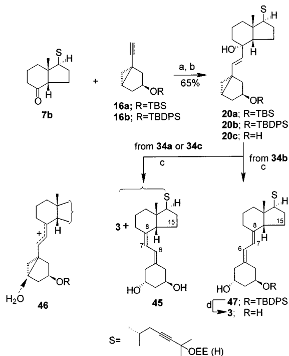
Scheme 6. (a) n BuLi, THF, -50 °C → room temp., 1 h; (b) [MeOCH 2 CH 2 O] 2 AlH 2 Na, Et 2 O, room temp., 12 h; (c) PTSA, dioxane/H 2 O (1:1), 63 °C, 3 h; (d) TBAF, THF, room temp.
